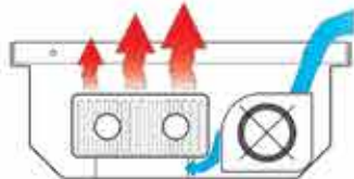
КОНВЕКТОР С ПРИНУДИТЕЛЬНОЙ КОНВЕКЦИЕЙ КВ, КVM, КVM2
