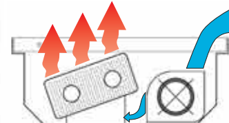
PLUS - ПОВЫШЕННОЙ ТЕПЛОПРОИЗВОДИТЕЛЬНОСТИ (С НАКЛОННЫМ ТЕПЛООБМЕННИКОМ)
